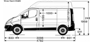
Vivaro Van L1 H1H&D2
