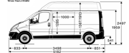
Vivaro Van L2 H1H&D2
